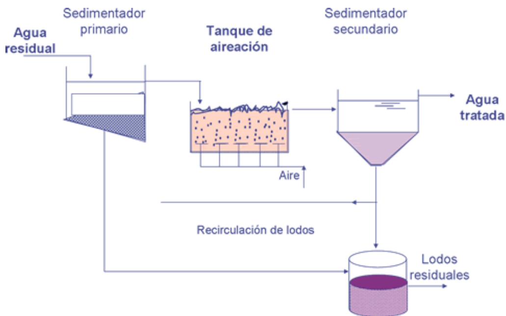
Figura N° 7 : Proceso planta de tratamiento mediante Lodos Activados
