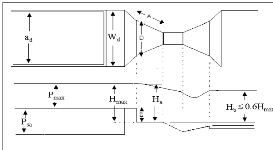
Figura N° 3 : Línea Piezometrica –Medidor Parshall
