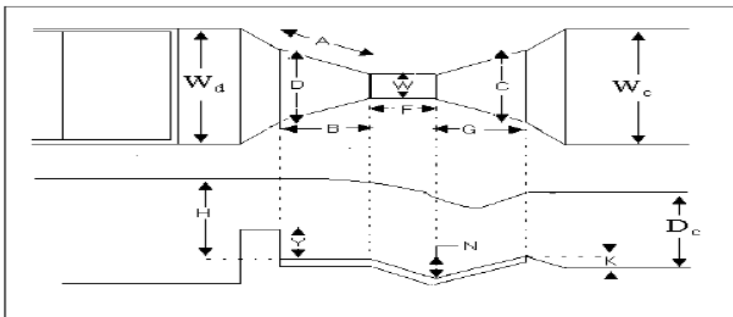
Figura N° 4 : Dimensionamiento del medidor Parshall
