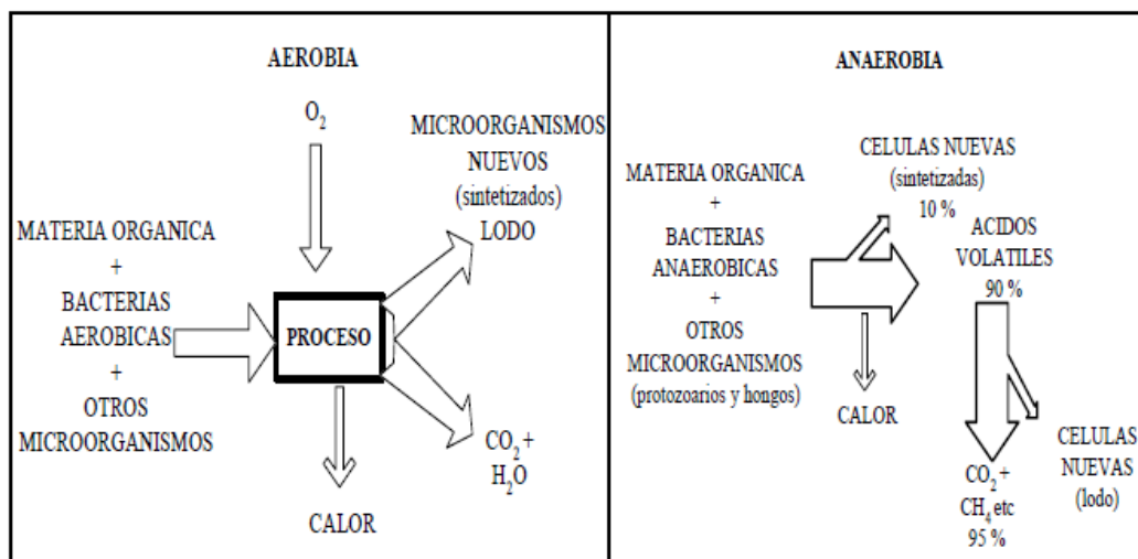
Figura N° 2 : Representación esquemática de los procesos de descomposición aerobios y anaerobios
