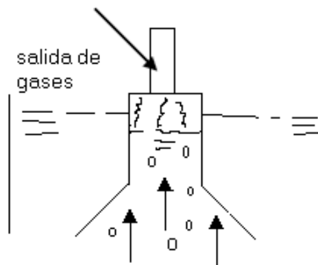
Figura N° 5 : Separador de gas líquido Sólido
