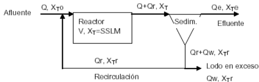
Figura N° 6 : Proceso Propuesto
