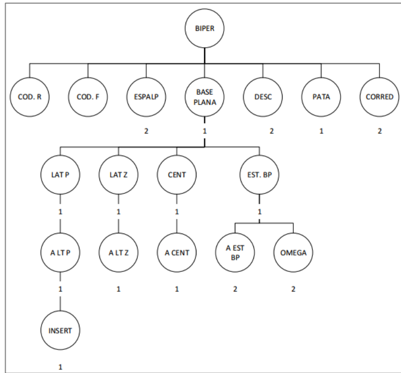
Ilustración 5 - Lista estructurada de materiales: Asiento Bipersonal
