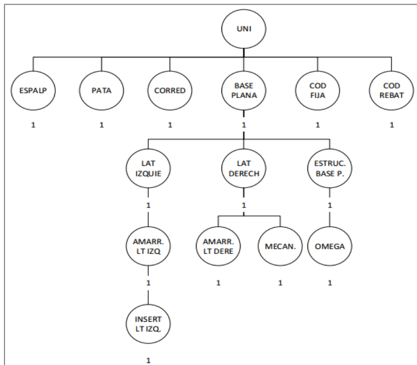
Ilustración 6 - Lista estructurada de materiales: Asiento Unipersonal
