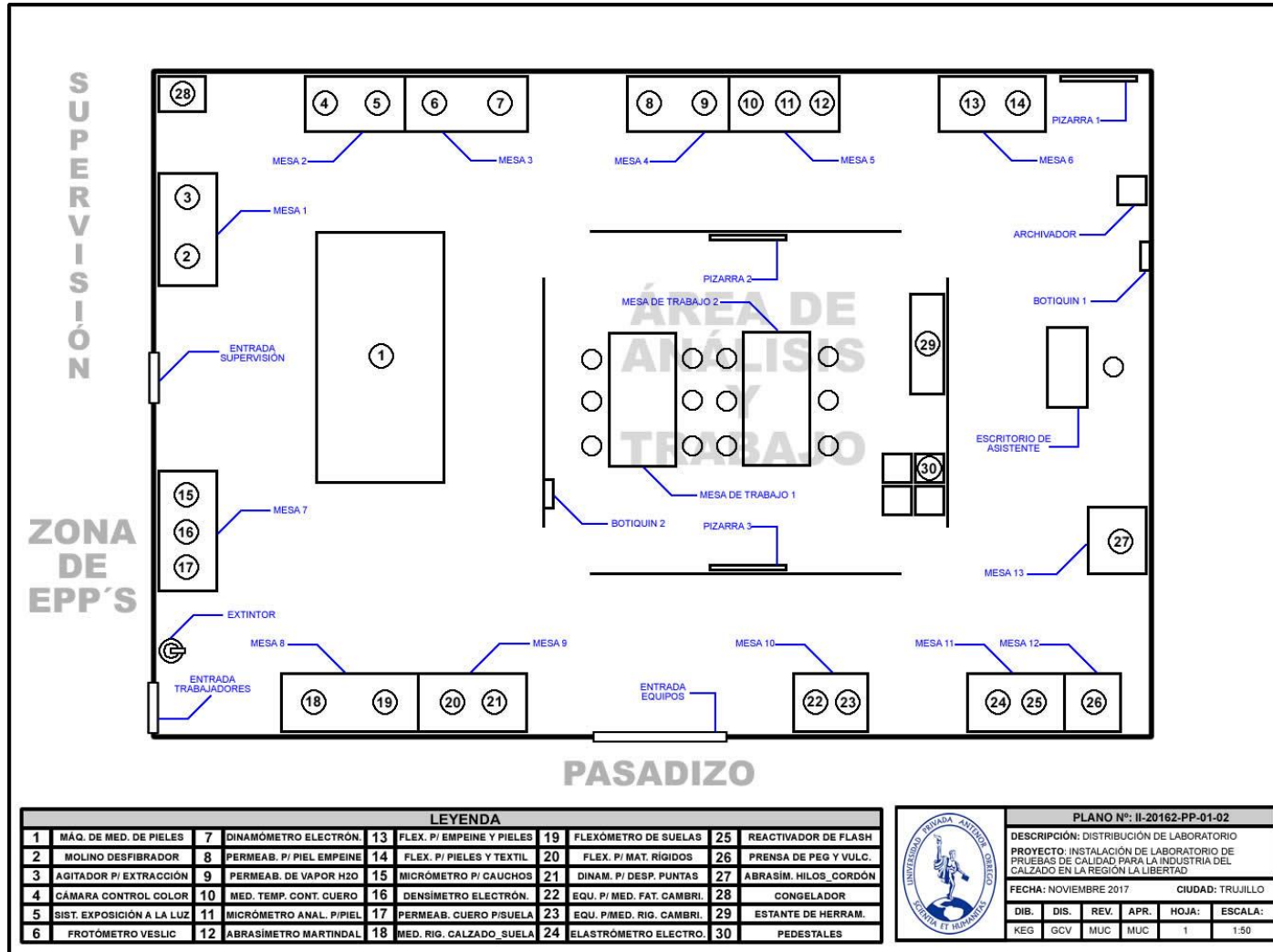
Figura 8. Plano del Laboratorio de Pruebas de Calidad
