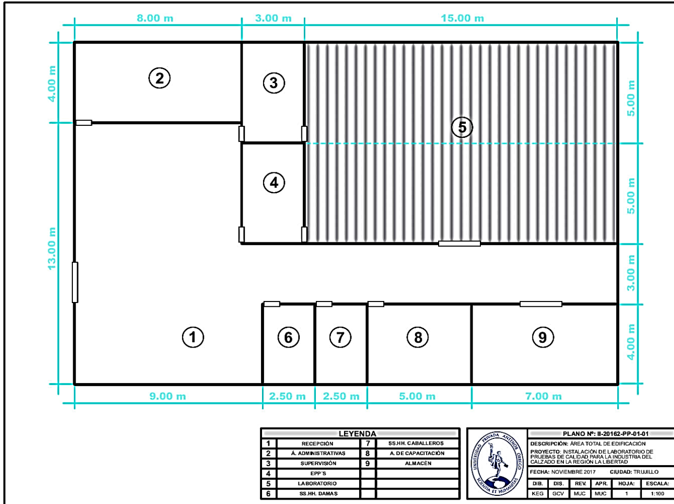
Figura 10. Plano de Edificación con Áreas Complementarias
