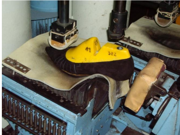
Figura 7. Máquina para Pegado de Suelas
