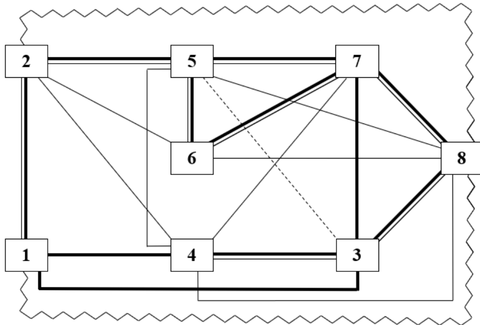
Gráfico 14. Diagrama Relacional óptimo de edificación
