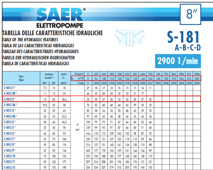
IMAGEN N° 27: Ficha Técnica Bomba Saer 20 HP S181C-2
