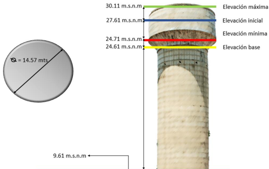
ESQUEMA N° 2: Reservorio Elevado
