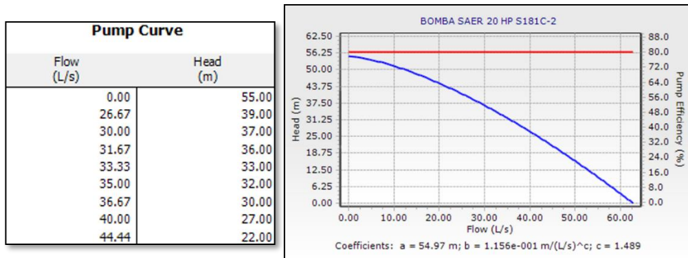
IMAGEN N° 28: Curva de Trabajo Bomba Saer 20 HP S181C-2
