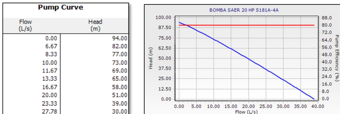
IMAGEN N° 22: Curva de Trabajo Bomba Saer 20 HP S181A-4A
