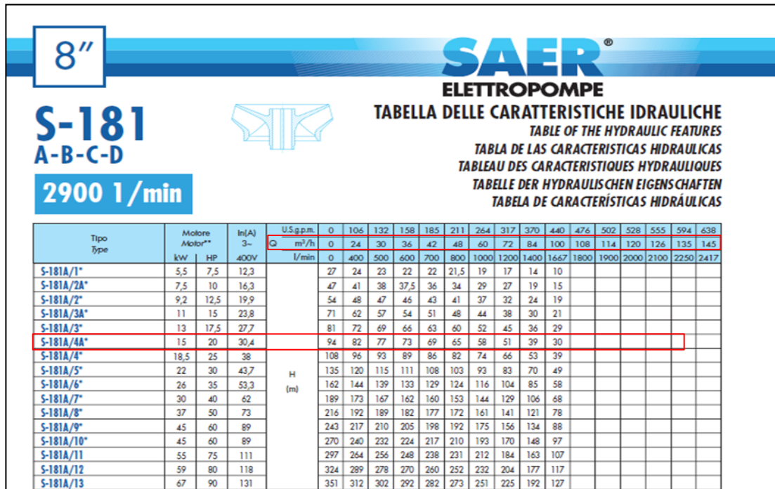
IMAGEN N° 21: Ficha Técnica Bomba Saer 20 HP S181A-4A
