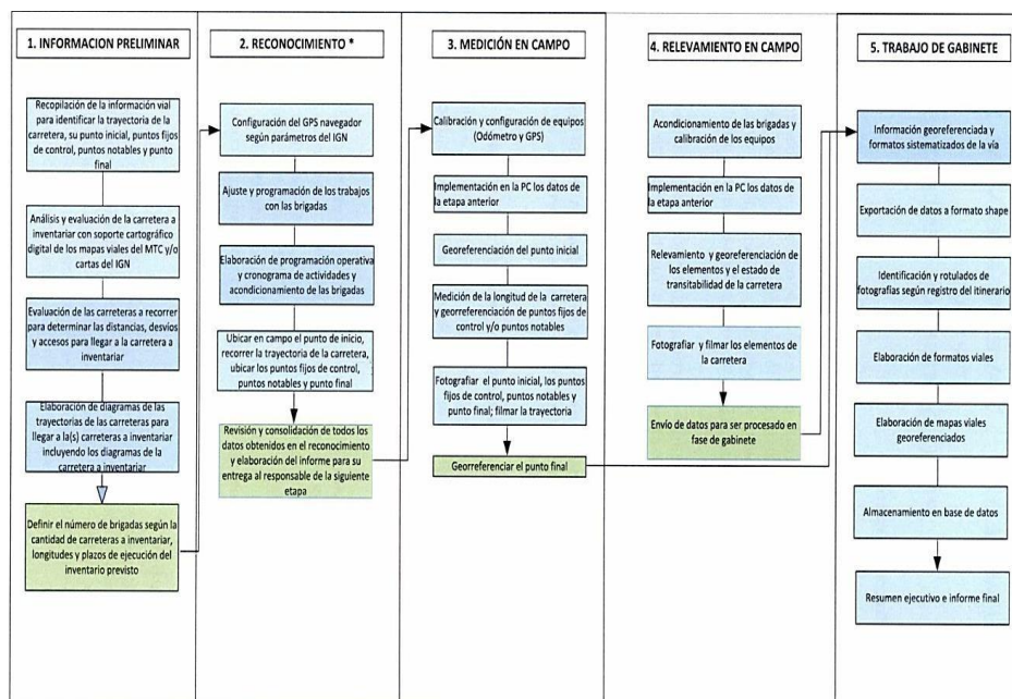
Descripción general del proceso del inventario vial básico
