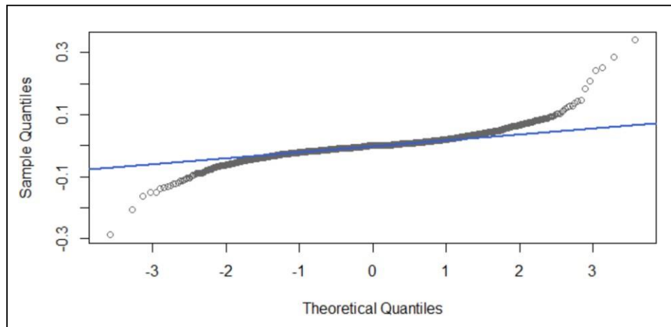
Figura 12: Diagrama Cuantil-Cuantil
